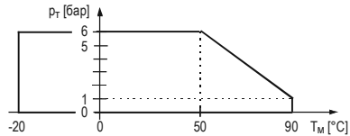
Давление p_T , выполняющее функции температуры T_M , для модели с фланцем PP
