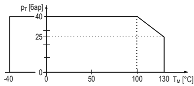
Давление p_T , выполняющее функции температуры T_M , для всех моделей (кроме модели с фланцем PP)
