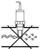
При установке на трубе зубья вилки должны быть параллельны направлению потока
