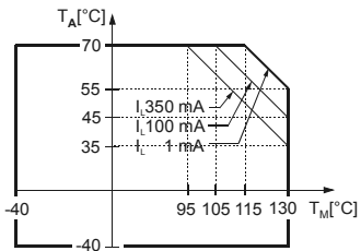
Предельные значения температуры для моделей постоянного тока, токовая нагрузка [IL]
