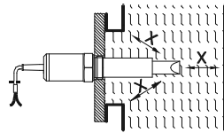
Модель с фланцем, предельное расстояние: x > 5 \text{ мм}
