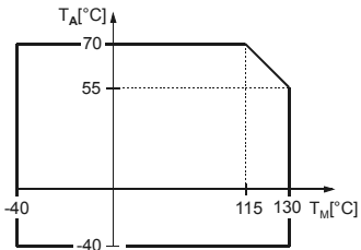
Предельные значения температуры для моделей постоянного тока, температура окружающей среды T_A и температура среды погружения T_M
