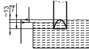
Точка переключения и разница значений переключения по воде при 25 °С
